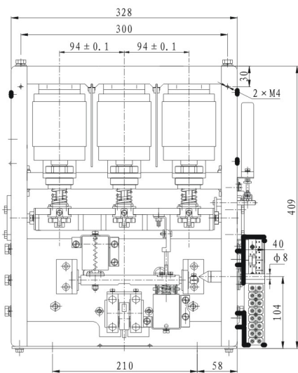
外形及安装尺寸图
